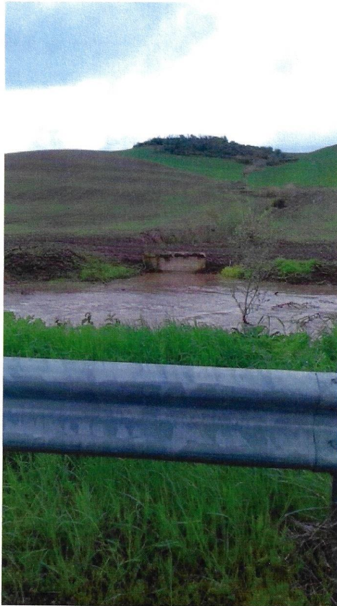
Foto scattata in data 15 aprile dalla s.p. ex n° 5 – Il livello idrico del torrente Locone impedisce il deflusso delle acque dell'affluente in foto con conseguente inondazione dei terreni limitrofi
